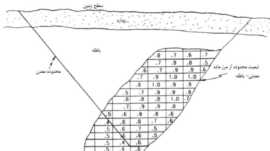
شکل ۴-۶- یک مقطع عرضی از معدن که یک دیواره و کف معدن در ماده معدنی قرار دارد.
