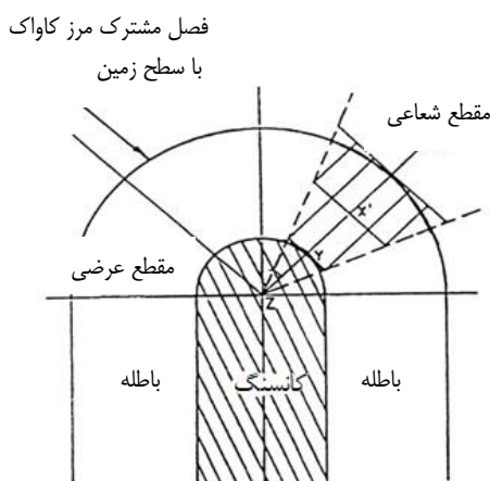
شکل ۴-۸- ناحیه تاثیر مقطع شعاعی
