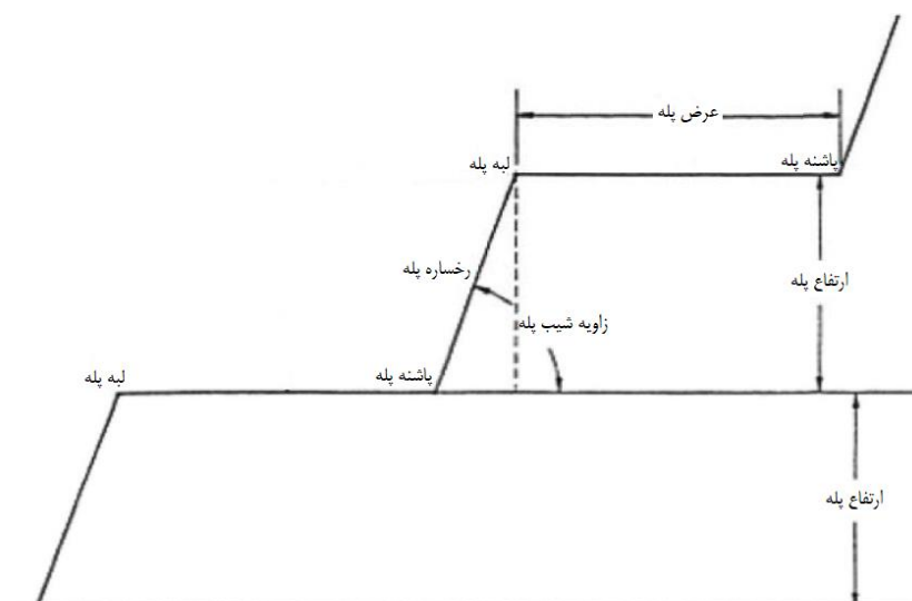
شکل ۱-۲- نمای از دو پله معدن
