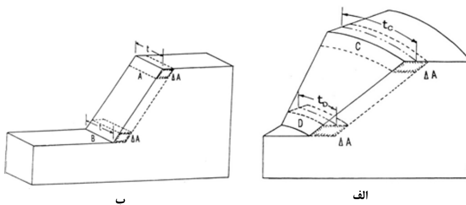
شکل ۴-۷- اختلاف مقاطع شعاعی و عرضی (الف- اختلاف حجم اجزا در کف و بالای مقاطع شعاعی. ب- یکسان بودن حجم اجزا در کف و بالای مقاطع عرضی)
