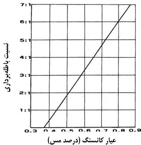
شکل ۴-۳- منحنی نسبت باطله برداری- عیار ماده معدنی
