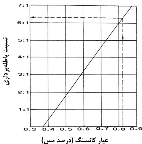
شکل ۴-۴- تعیین نسبت باطله برداری سربه سری برای گزینه G_1
