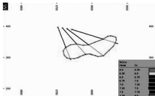
شکل ۲-۴- نمونه‌ای از رشته ایجاد شده برای تعیین مرز کانسار در یک مقطع
