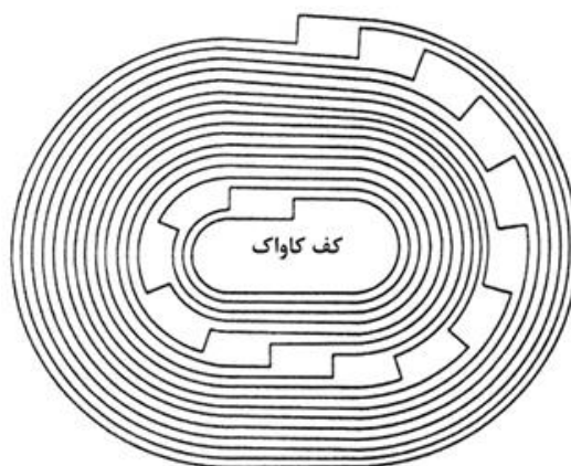
۴-۳۵- پلان مرکب کاواک پس از اضافه کردن رمپ
